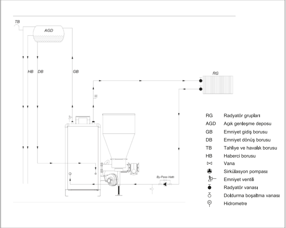
Şekil 3 – Tesisat Şeması EKO EKS 25-...-60
